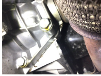
Ön aks, Aks mili, sağ > Yağ Kaçığı
